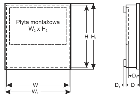
Konstrukcja natynkowa
